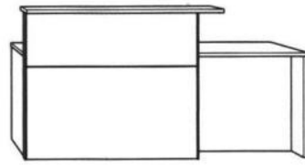
DZ89 2020*900*1075
