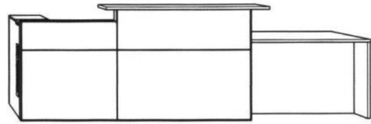
DZ80 3300*900*1075
